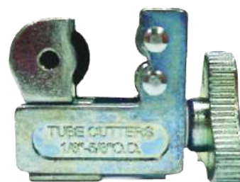
COD. CT-127 Tagliatubi 3-16mm Tagliatubi 1/8" - 5/8" Pipe cutter 3-16mm Pipe cutter 1/8" - 5/8"
